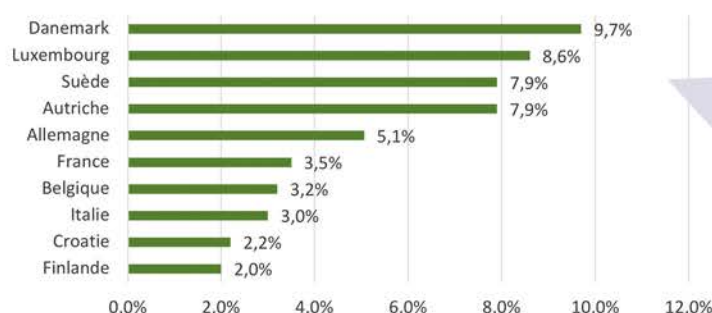
Figure 3 : les pays européens avec la plus grande part de marché bio en 2016 (%) (Eurostat, 2018)
